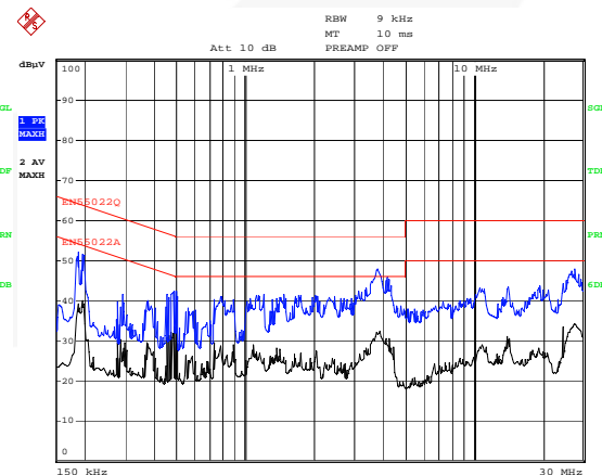
Figure 20. N: 230 / 50Hz
